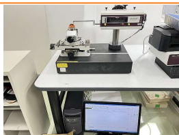
輪郭形状測定機 ミットヨ CV-2000 https://www.kkmt.co.jp/tools/156850 番号:C171275
